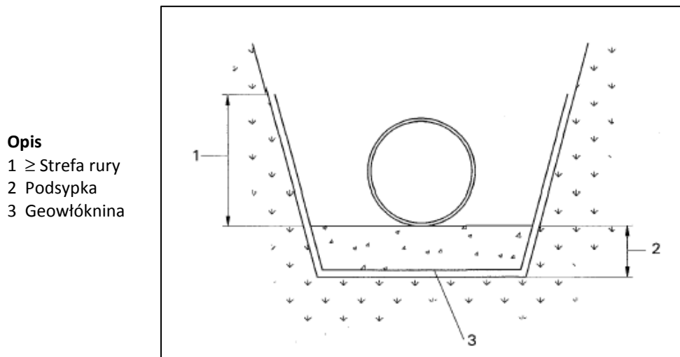
Rysunek 6. Zabezpieczenie przed migracją cząstek materiału gruntowego
