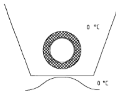
Rysunek 4. Izolacja termiczna z zastosowaniem otulin styropianowych
