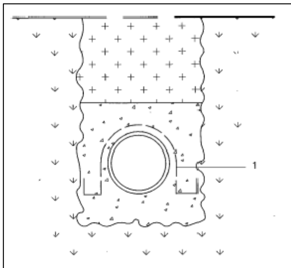
Rysunek 7. Geowłóknina jako zakotwienie zabezpieczające przed wypieraniem wód gruntowych wg PN-ENV 1046
