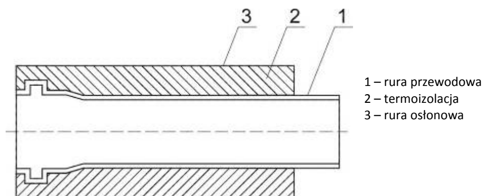
Rysunek 5. Rura kanalizacyjna PVC-U termoizolowana
