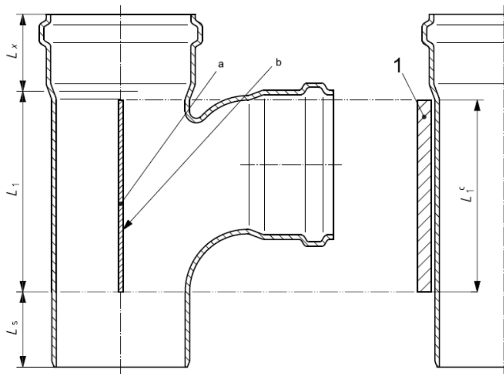
Rysunek 2. Wyznaczanie długości obliczeniowej dla trójnika
