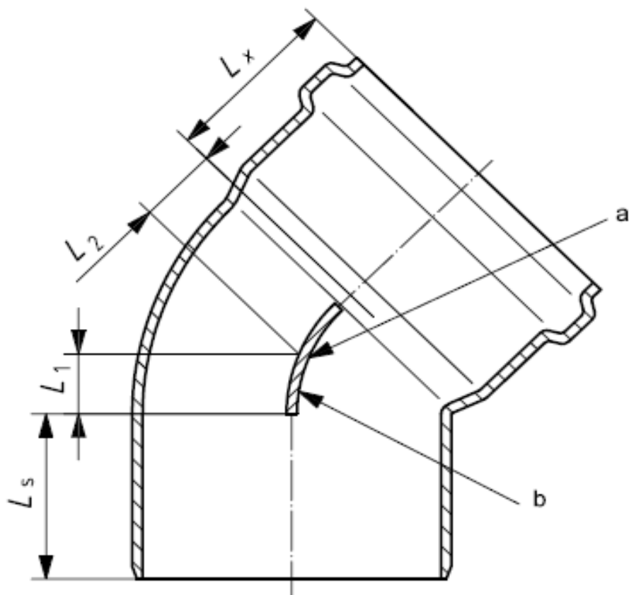
Rysunek 1. Wyznaczanie długości obliczeniowej dla kolana
